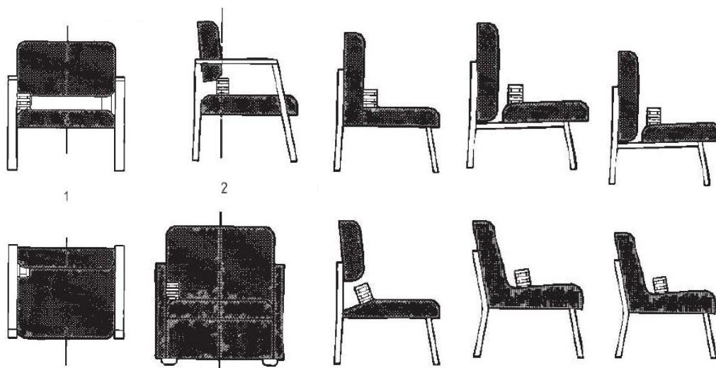
图 C.2 沙发和软包椅木垛放置位置示意图
