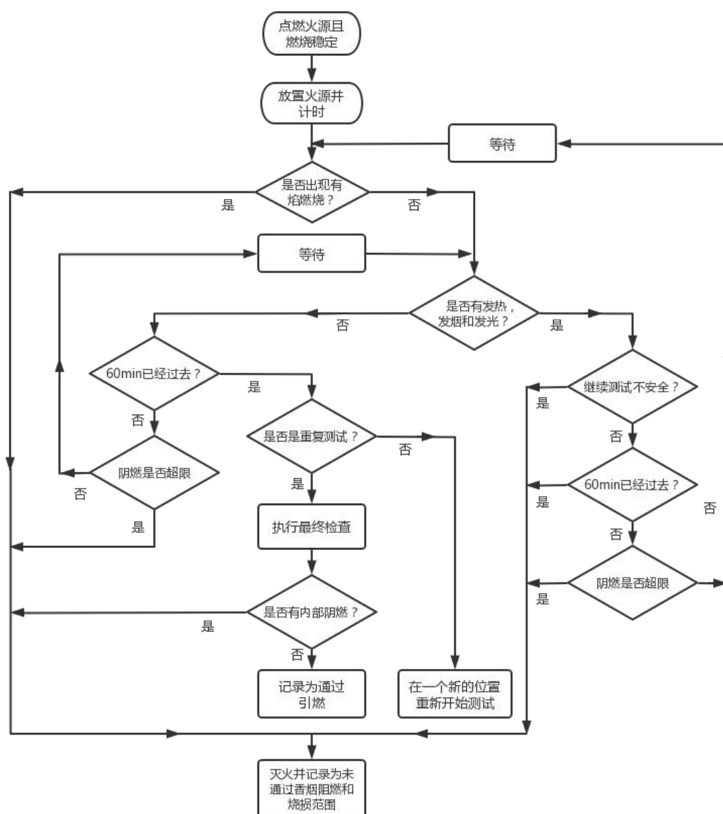
图 A.1 香烟引燃流程图
